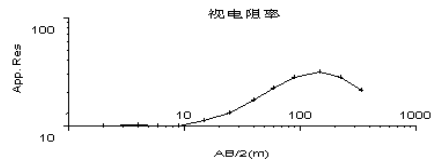
剖面 demo 上测深点s1 观测数据
